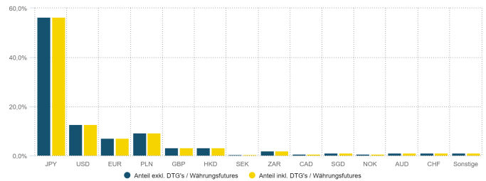
Währungsrisiko per 30.06.2024
